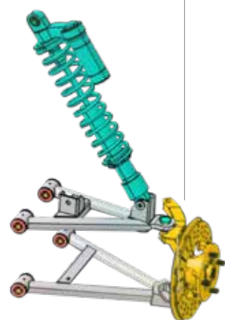
EINZELRAUFGÄNGUNG mit Doppelquerlenker Federweg 190 mm vorne, 210 mm hinten
